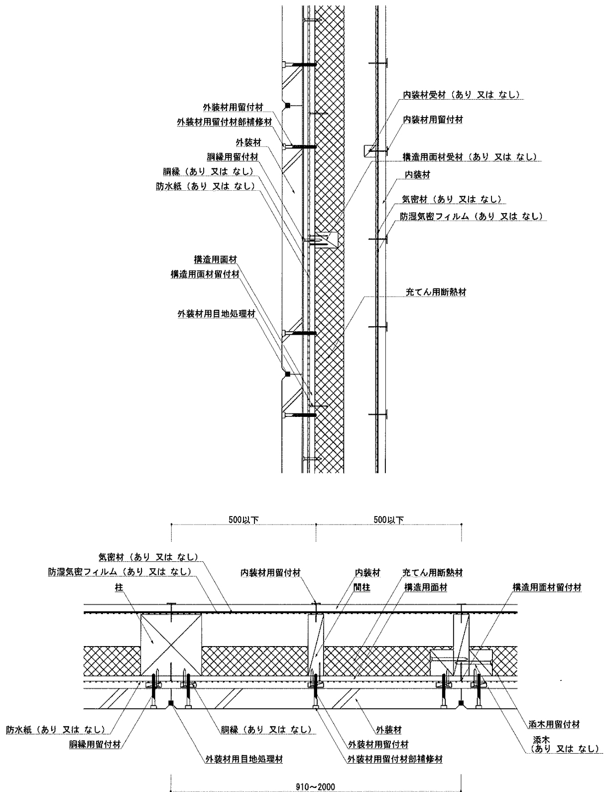
図2 構造説明図(水平垂直断面詳細図・内装材単張り)
