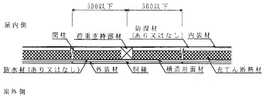
水平断面図
