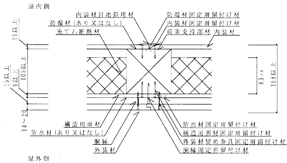
水平断面図詳細図
