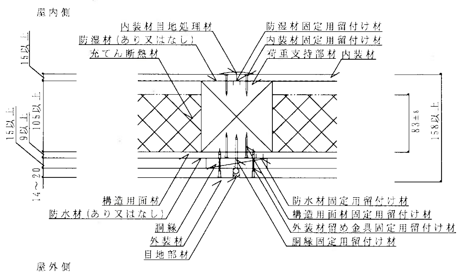
水平断面図詳細図
