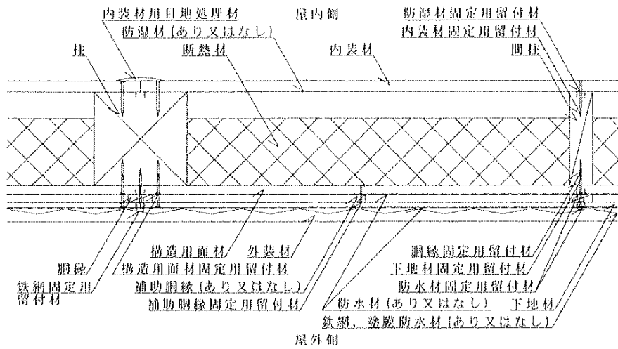
水平断面詳細図
