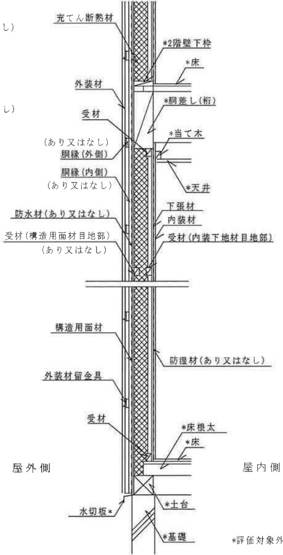
鉛直断面図
