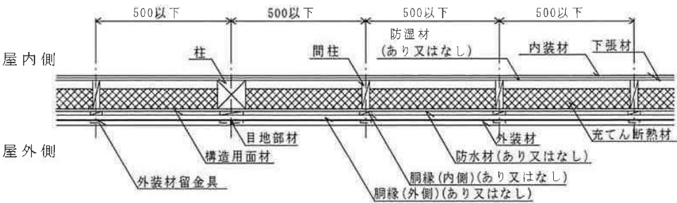
水平断面図
