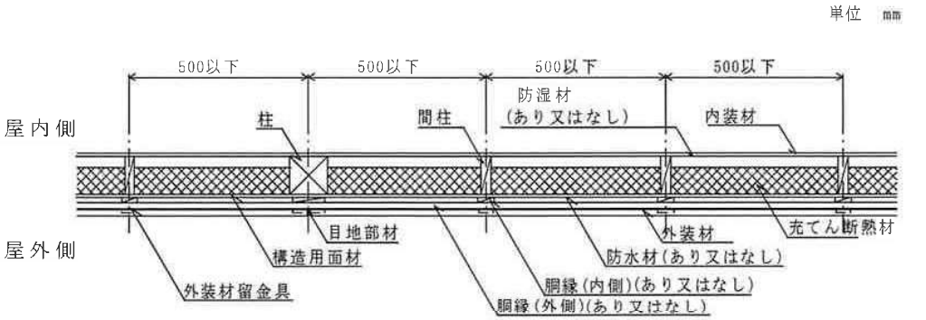
水平断面図
