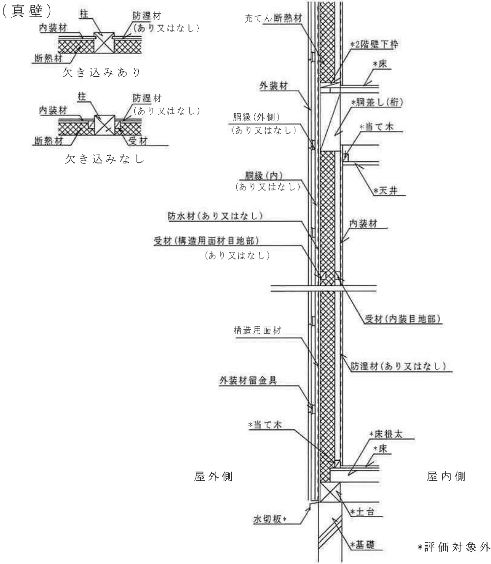
鉛直断面図
