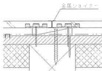
(3)金属ジョイナー目地 2)H形、T形
