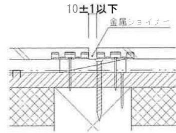
(3)金属ジョイナー目地
