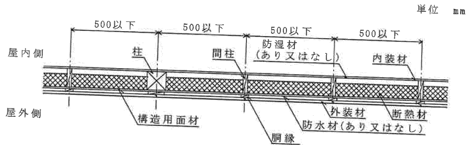
水平断面図
