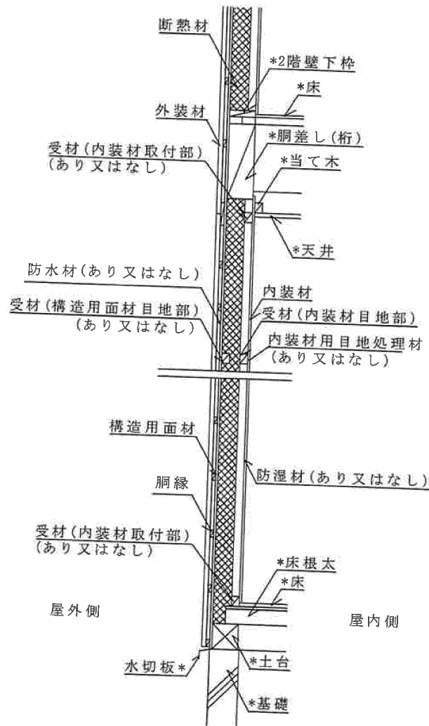
鉛直断面図
