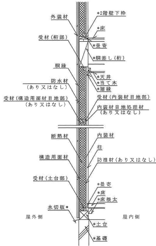
鉛直断面図 真壁造(柱欠き込み) 構造用面材あり 外装材：横張・縦胴縁
