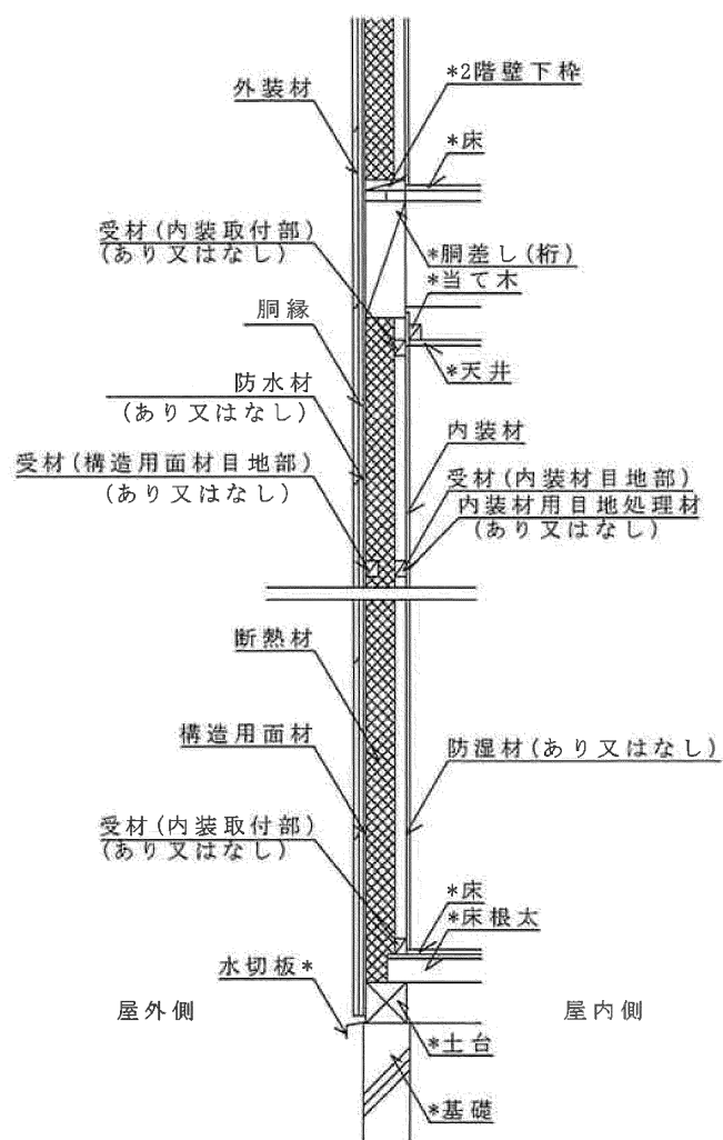
鉛直断面図 大壁造 構造用面材あり 外装材：横張・縦胴縁
