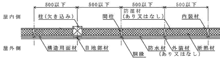
水平断面図
