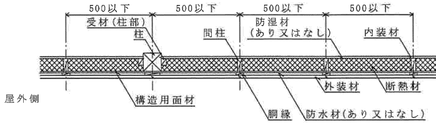
水平断面図
