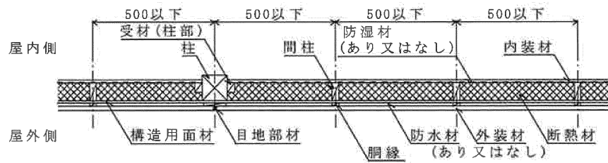
水平断面図
