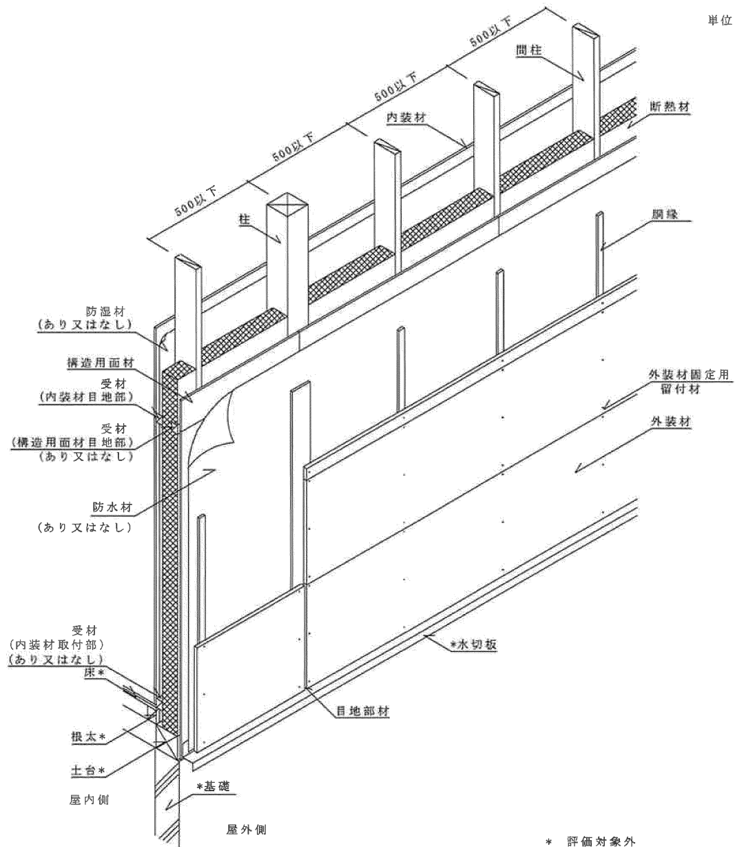
透視図 大壁造 構造用面材あり 外装材：横張・縦胴縁
