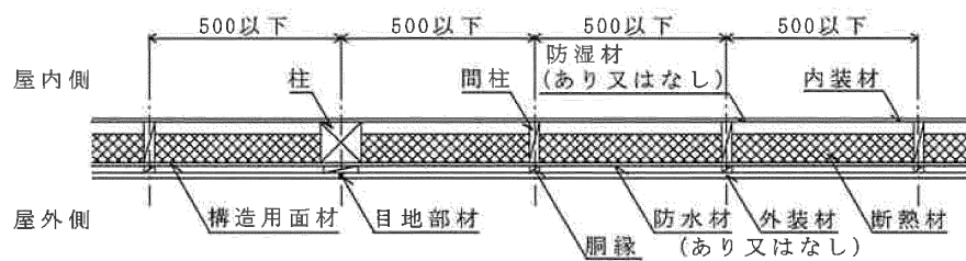
水平断面図
