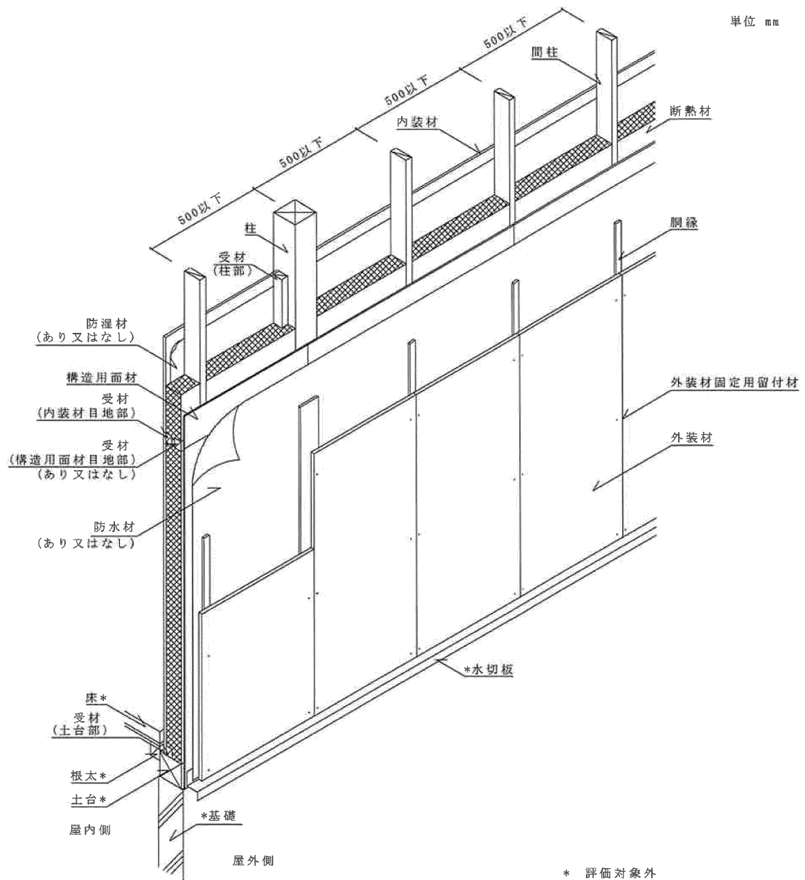
透視図
