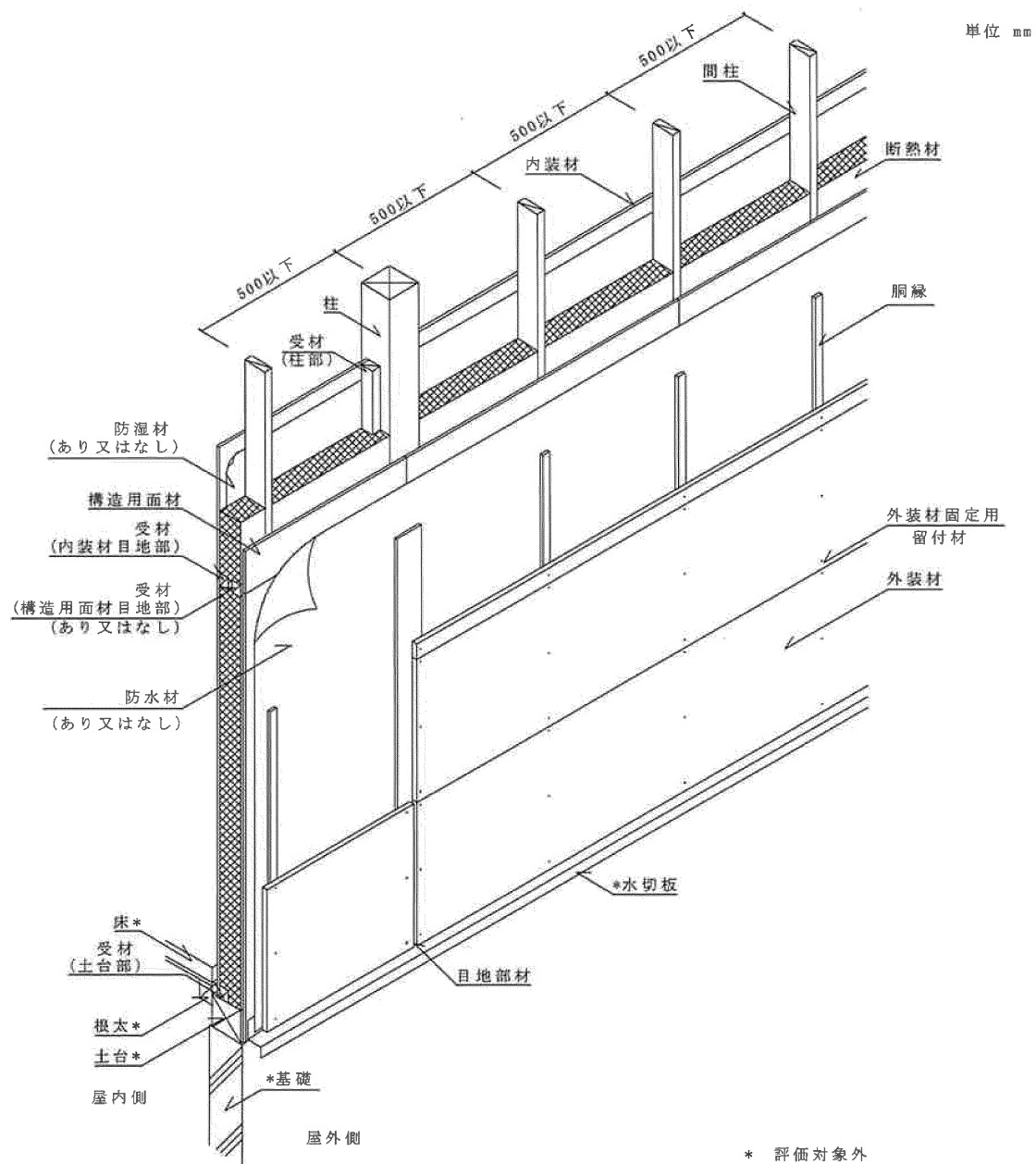
透視図
