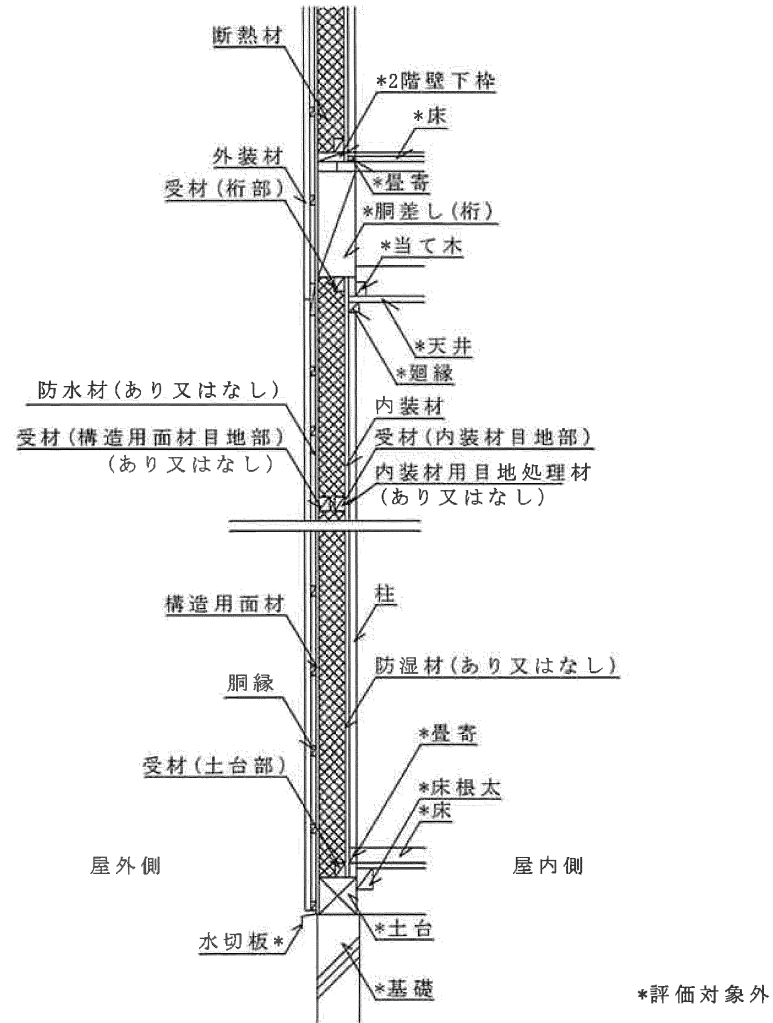
鉛直断面図
