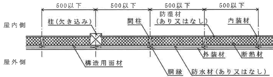
水平断面図
