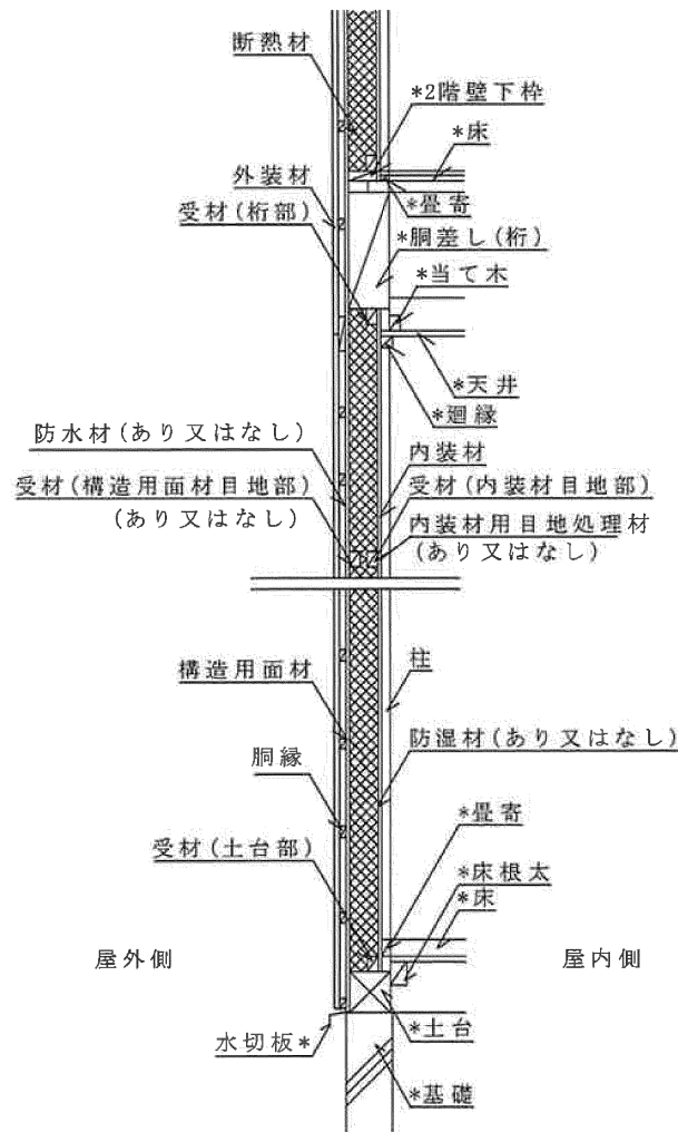
鉛直断面図
