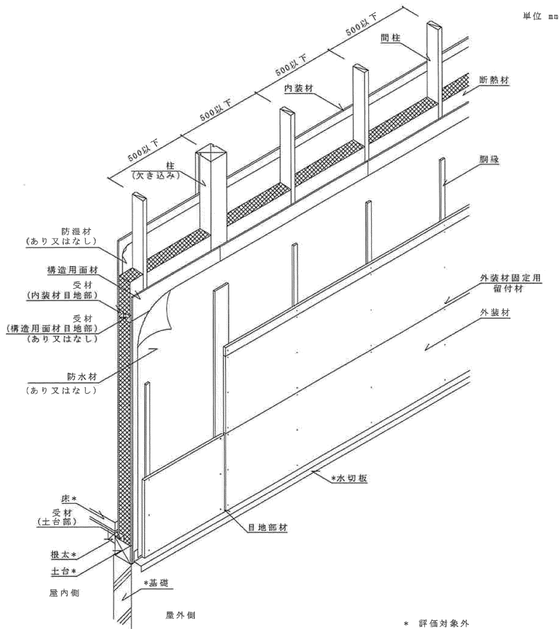
透視図 真壁造(柱欠き込み) 構造用面材あり 外装材：横張・縦胴縁
