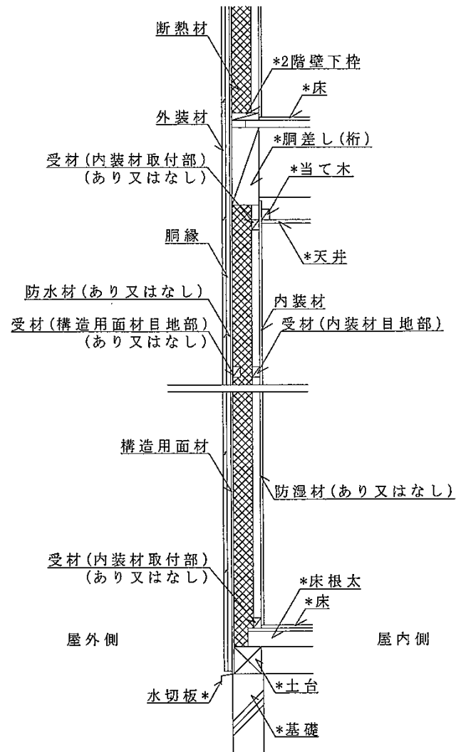
鉛直断面図
