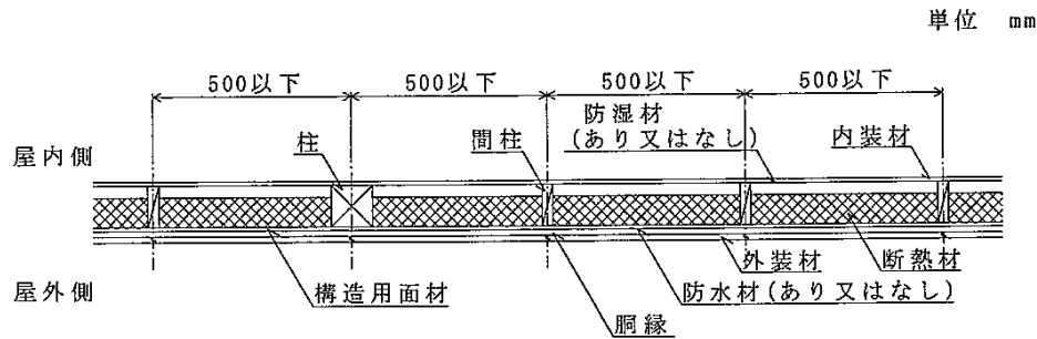
水平断面図
