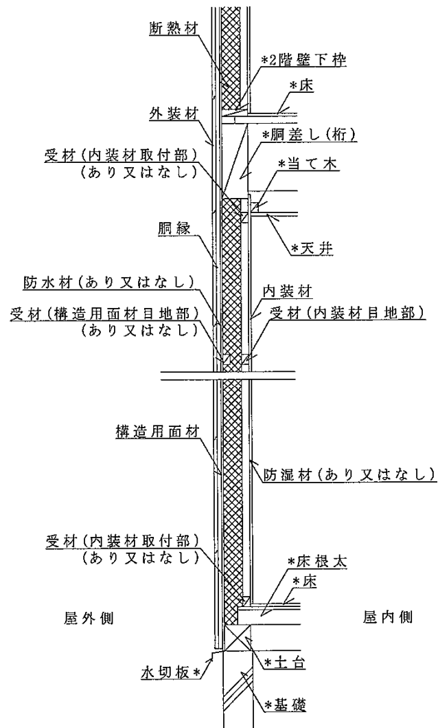
鉛直断面図
