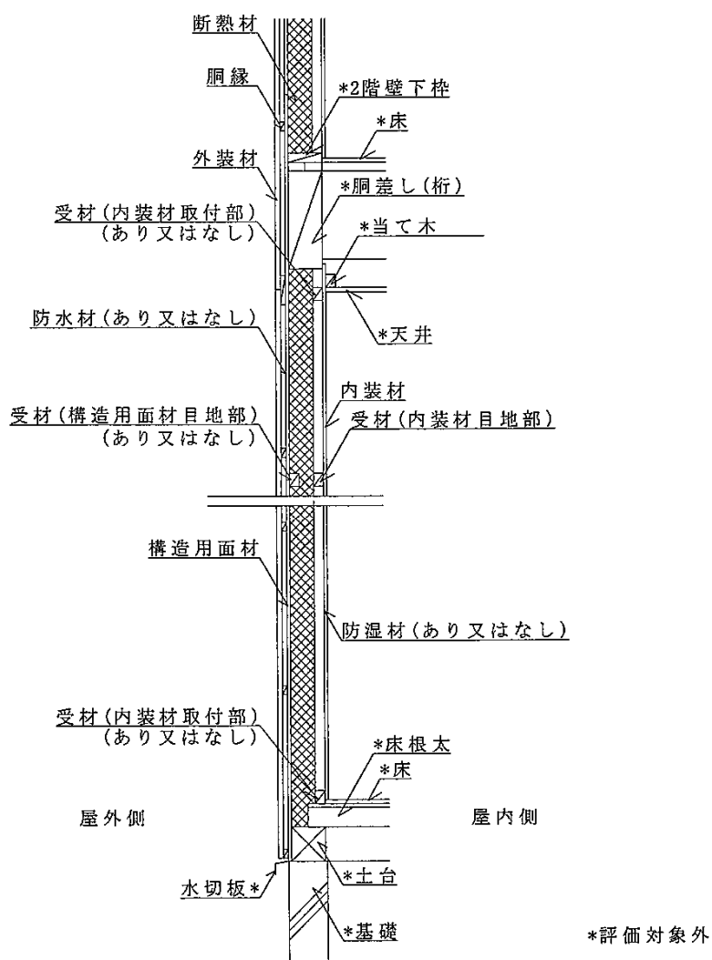
鉛直断面図
