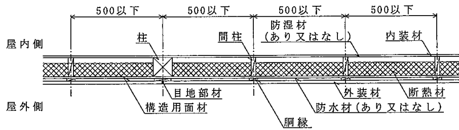
水平断面図
