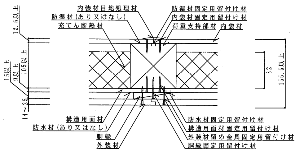
水平断面図
