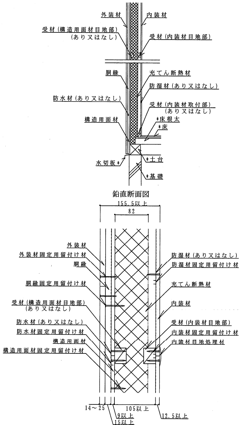
鉛直断面図詳細図
