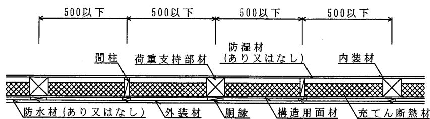
水平断面図
