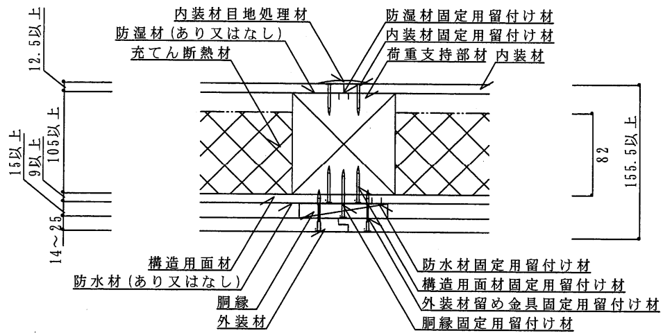
水平断面図詳細図
