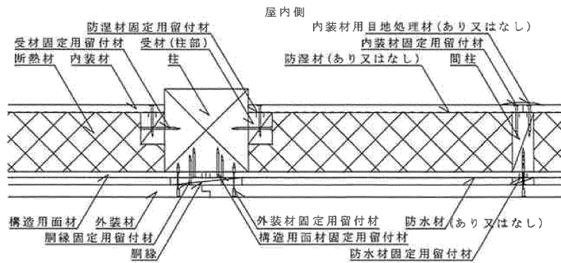
水平断面詳細図
