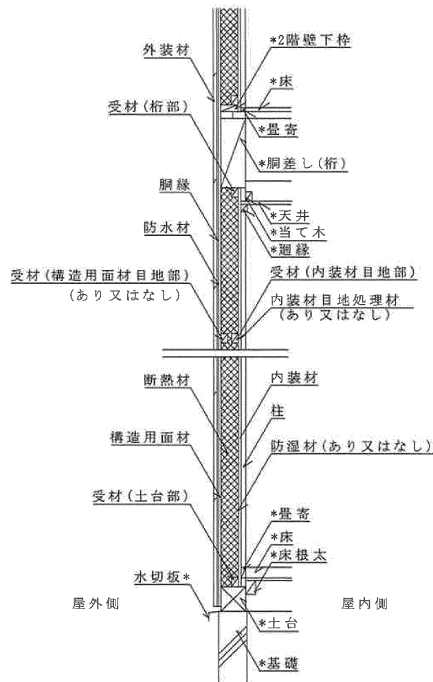
鉛直断面図 真壁造(柱部受材) 構造用面材あり
