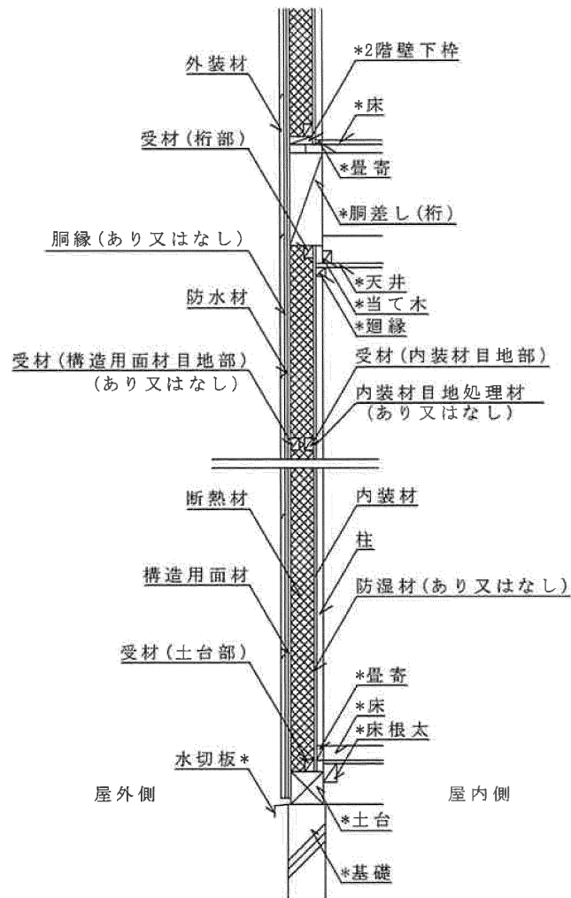
鉛直断面図 真壁造(柱欠き込み) 構造用面材あり
