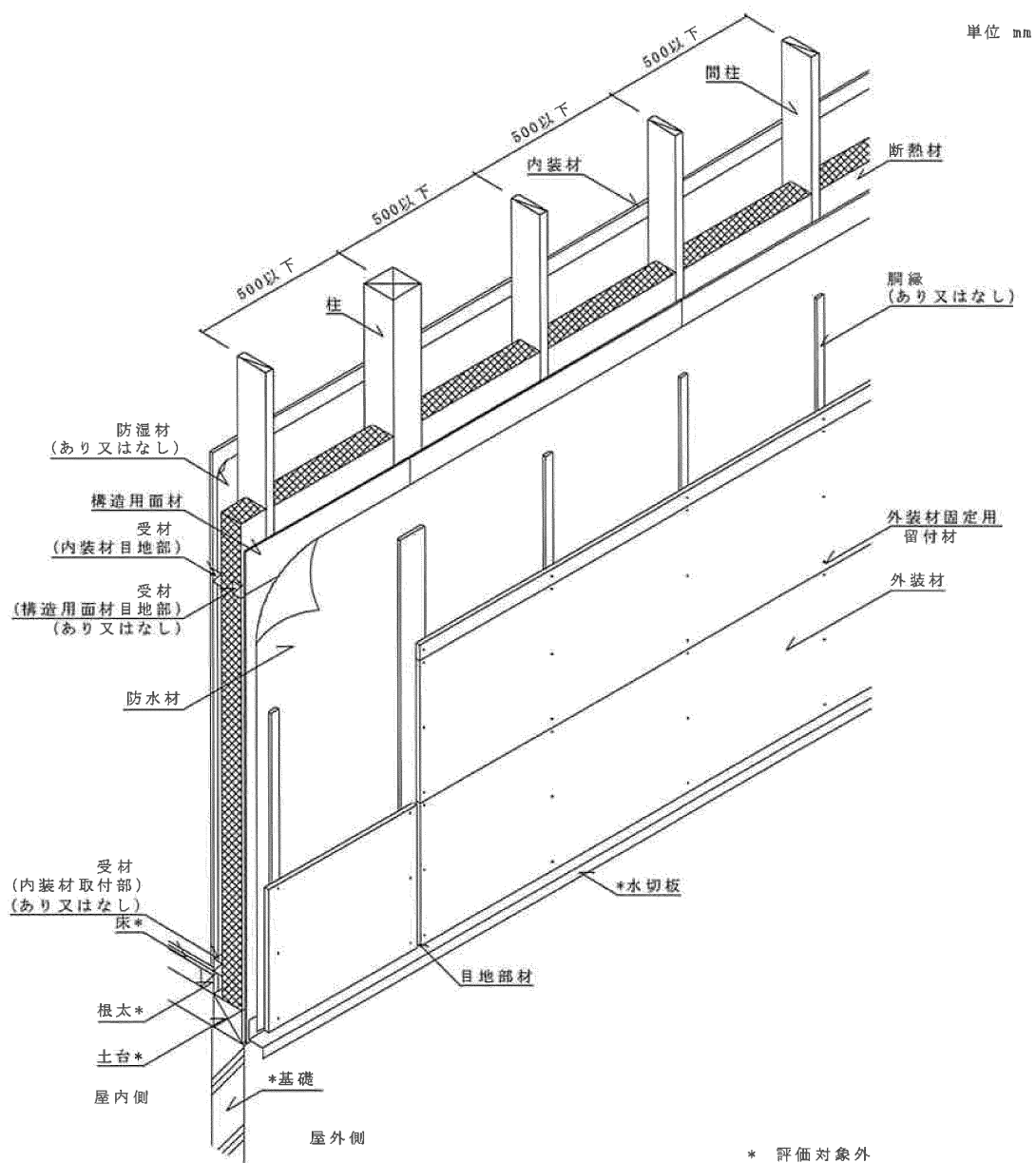
透視図 大壁造 構造用面材あり
