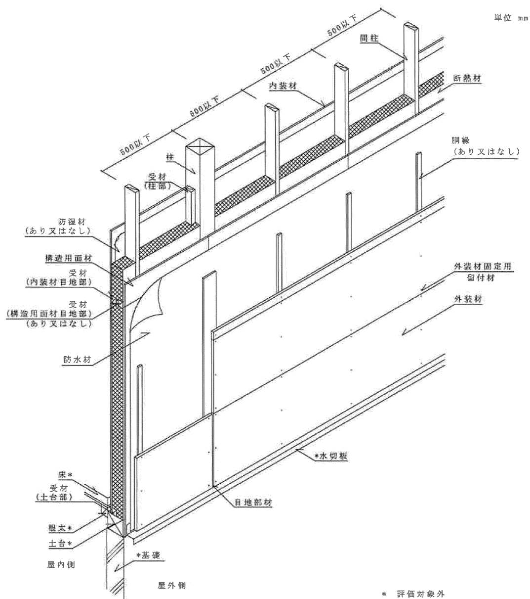
透視図 真壁造(柱部受材) 構造用面材あり
