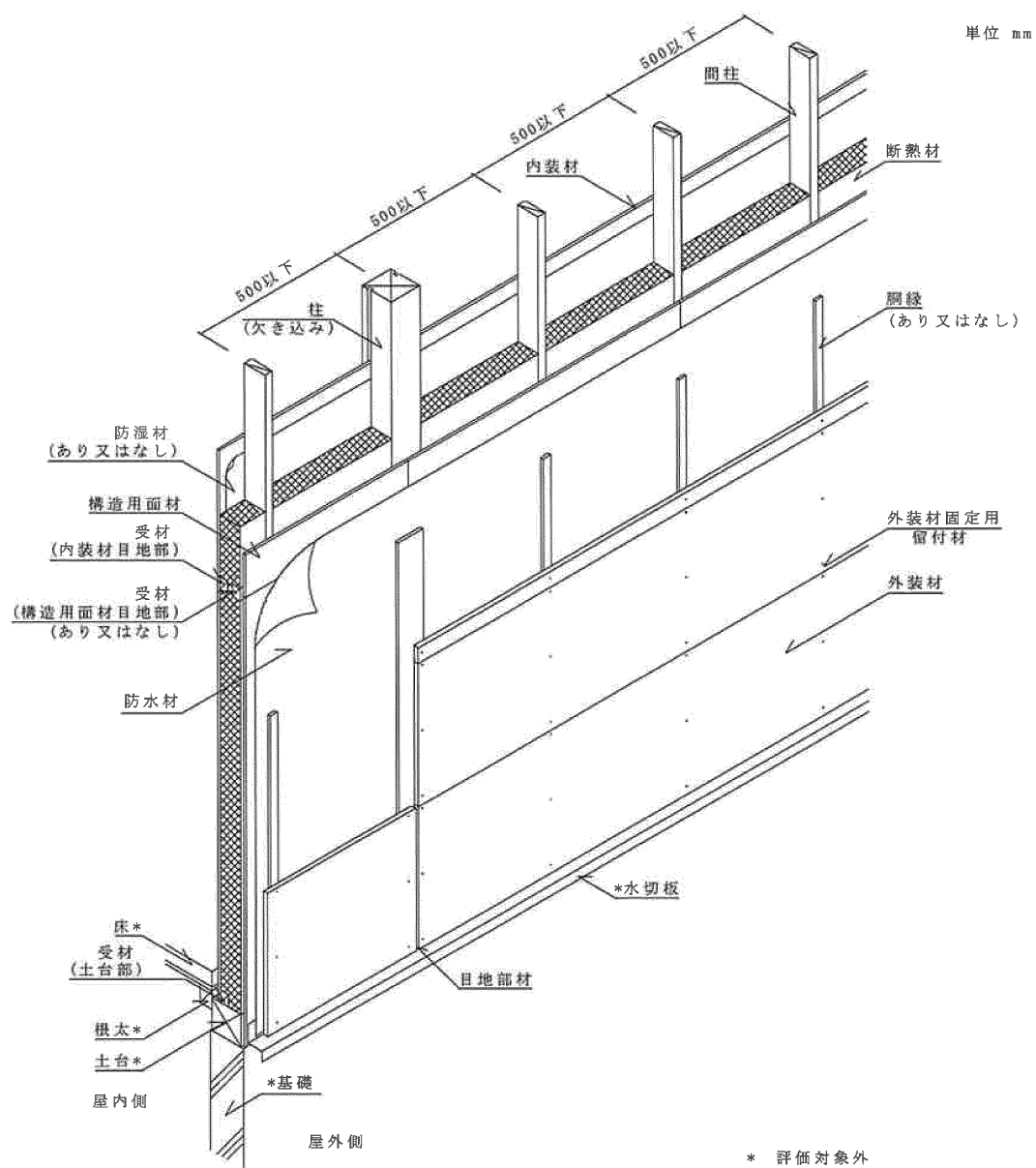
透視図 真壁造(柱欠き込み) 構造用面材あり
