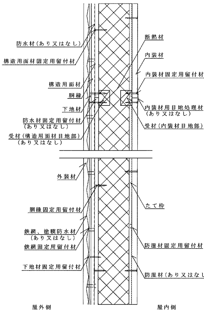
鉛直断面詳細図 複層下地工法・通気層あり
