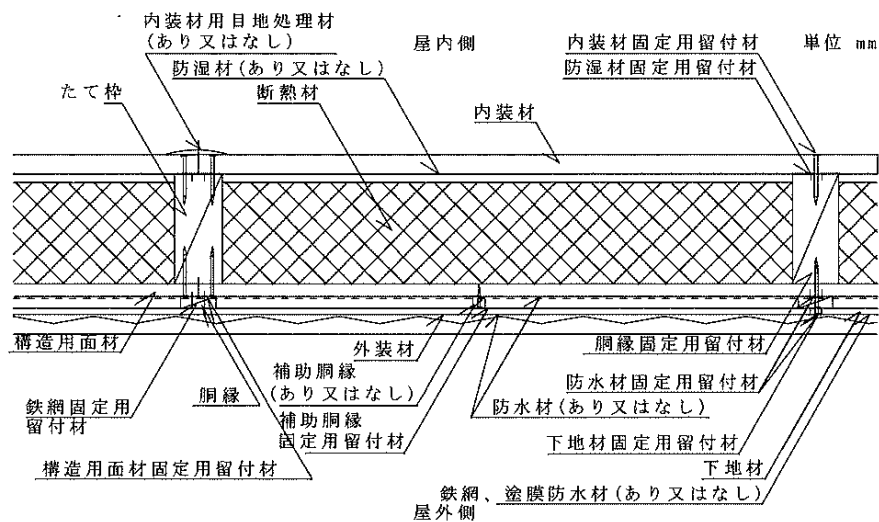
水平断面詳細図
