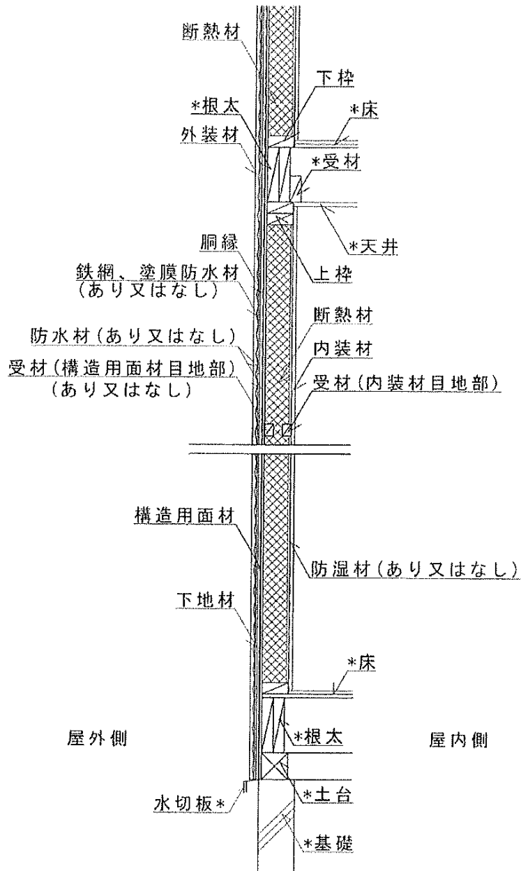
鉛直断面図 複層下地工法・通気層あり
