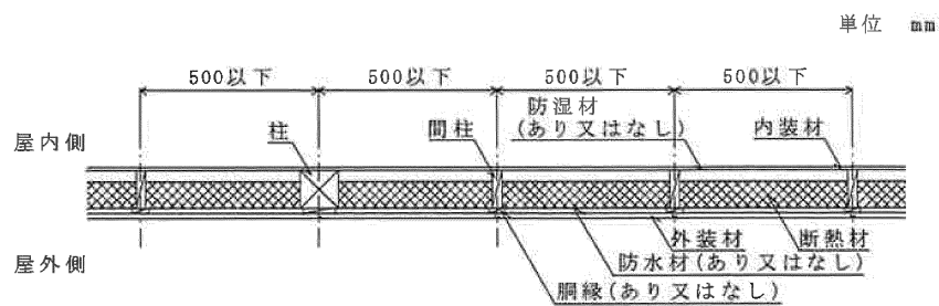
水平断面図
