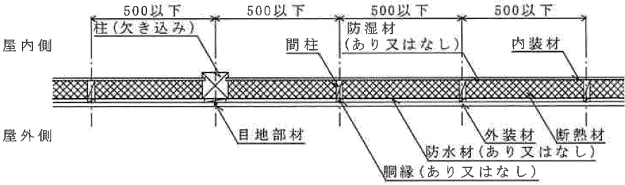
水平断面図
