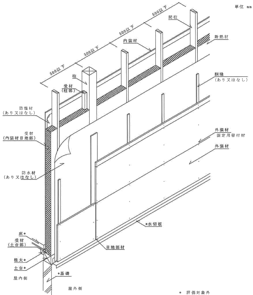
透視図 真壁造(柱部受材) 構造用面材なし
