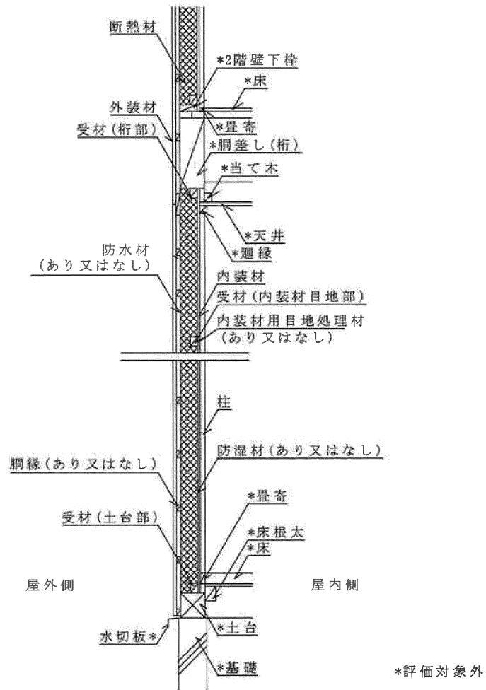
鉛直断面図
