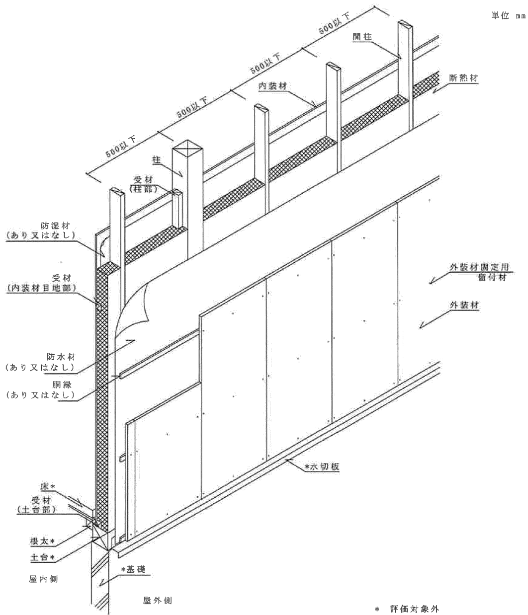
透視図
