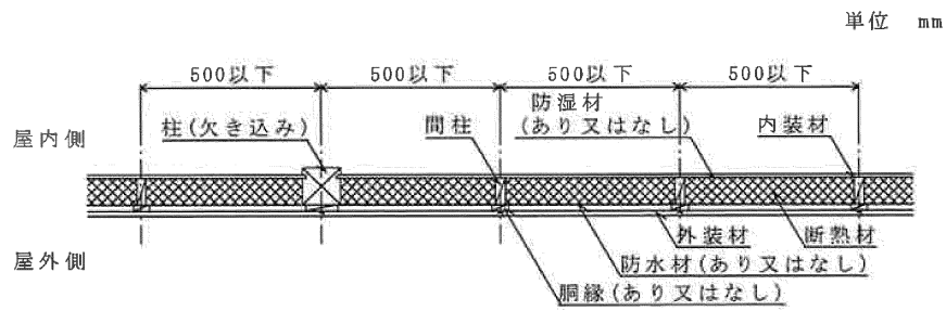
水平断面図
