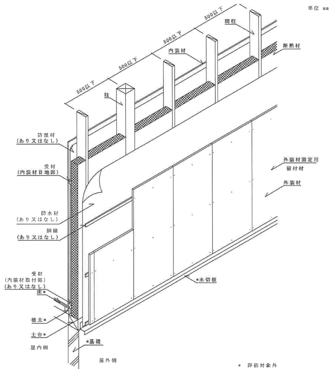
透視図 大壁造 構造用面材なし 外装材：縦張・横胴縁
