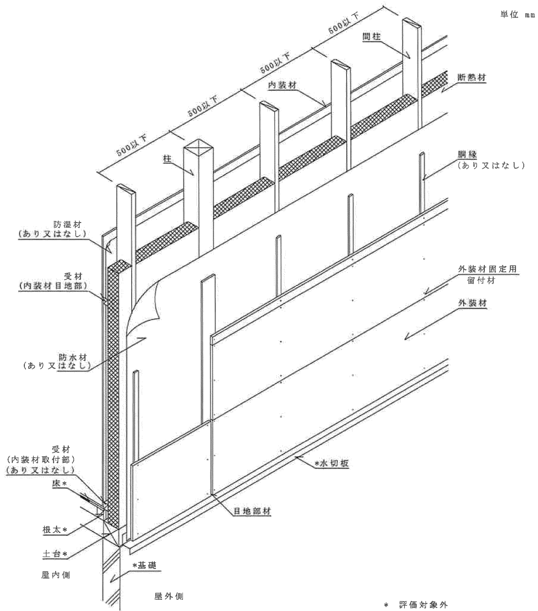
透視図 大壁造 構造用面材なし
