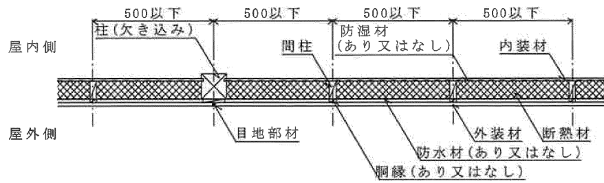
水平断面図
