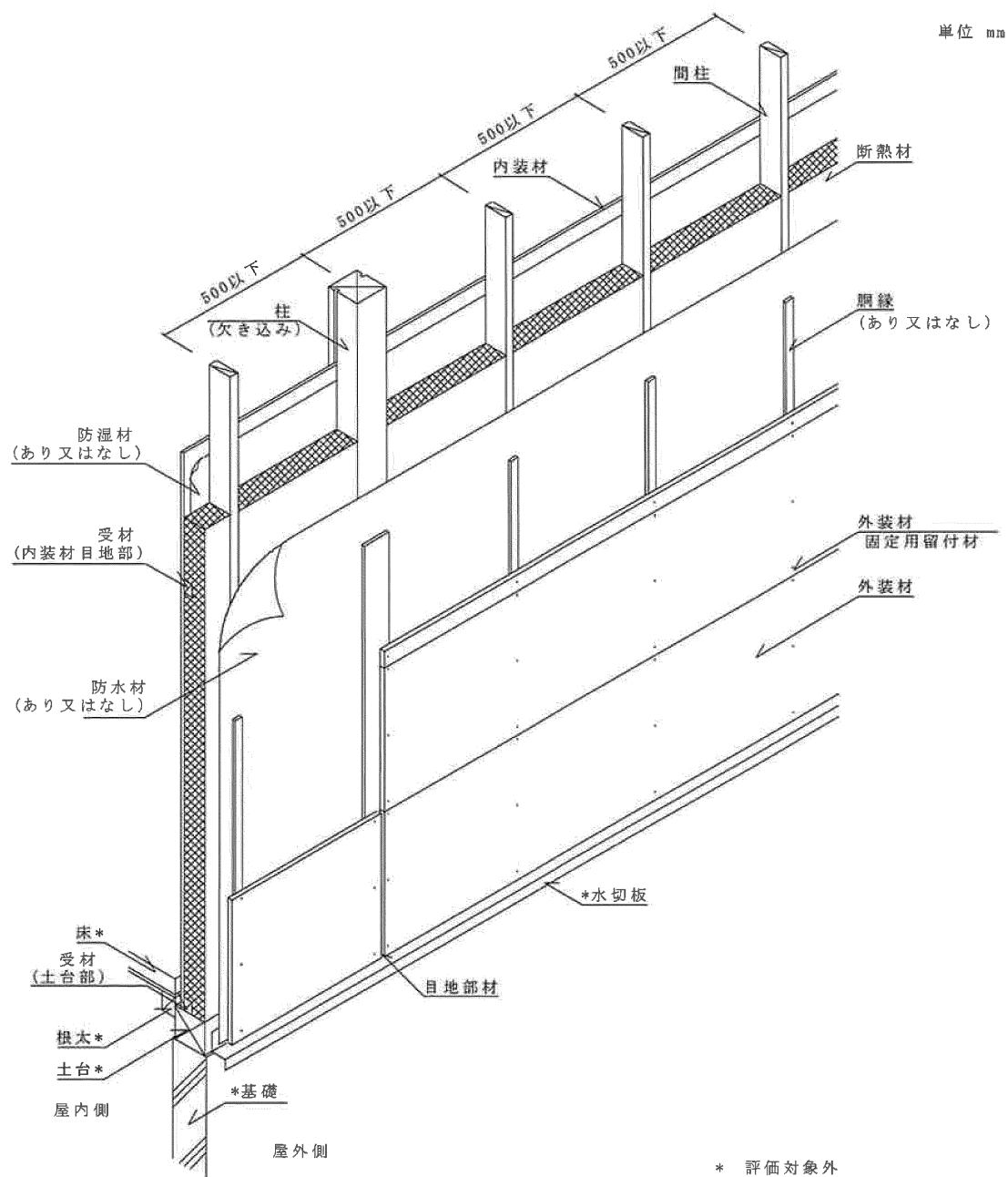
透視図 真壁造(柱欠き込み) 構造用面材なし
