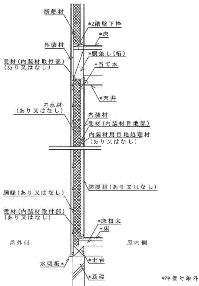
鉛直断面図
