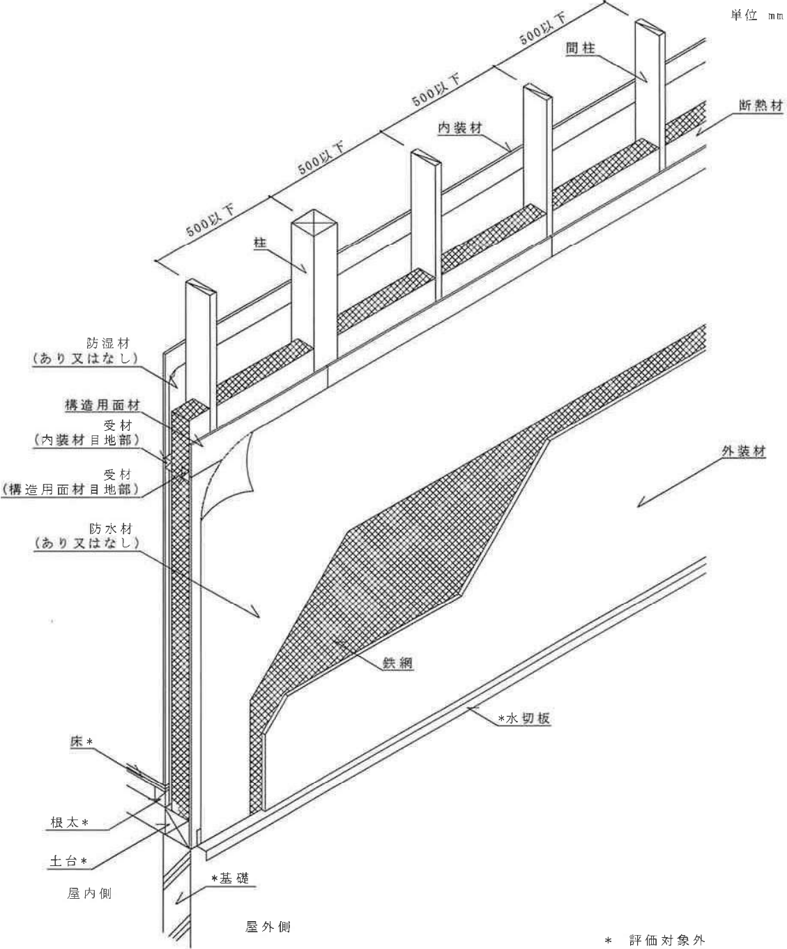
透視図 大壁造/直張仕様 構造用面材あり・下地材なし
