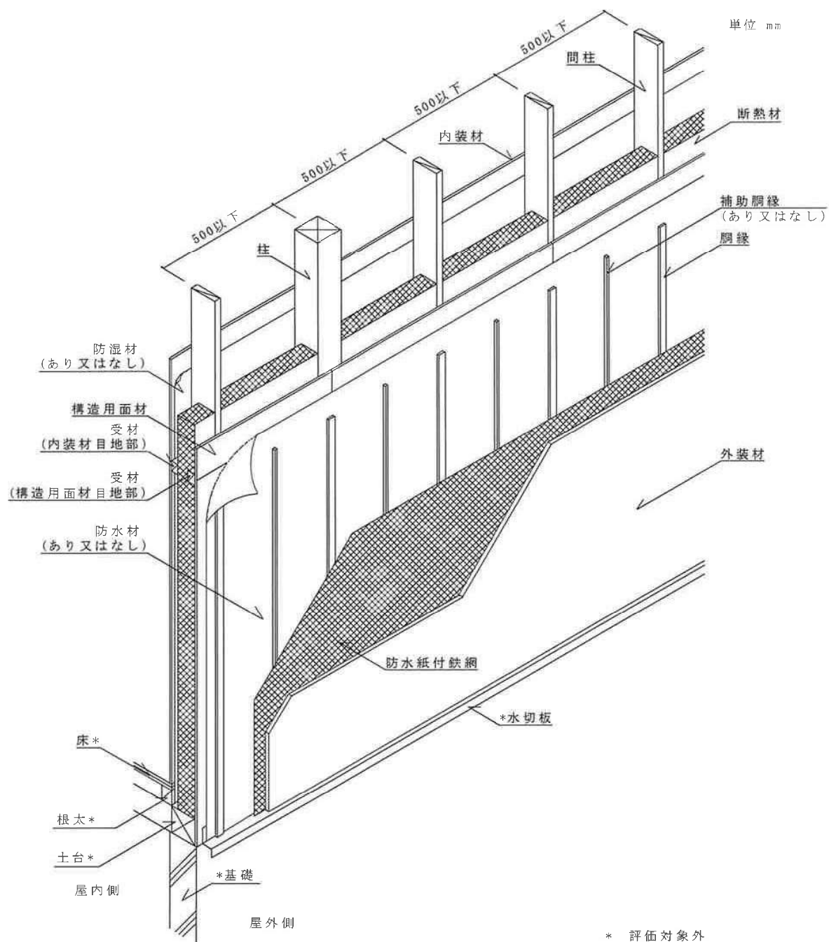
透視図
