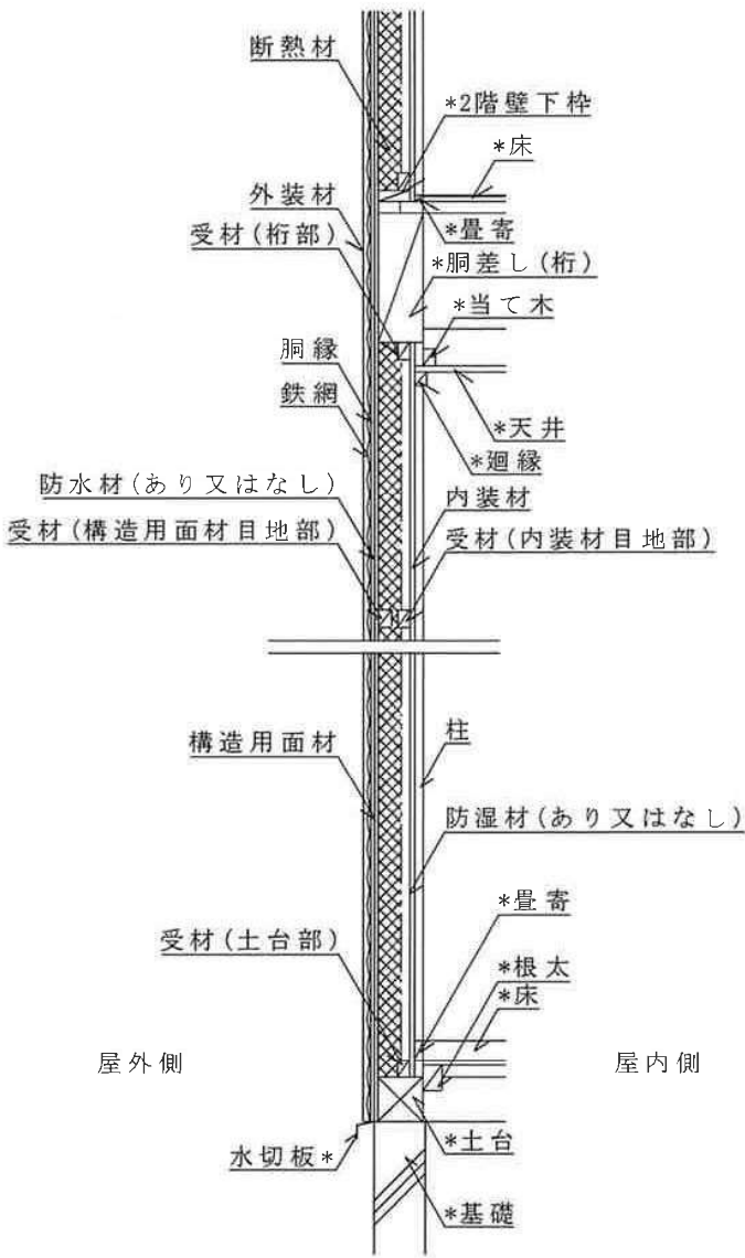
鉛直断面図
