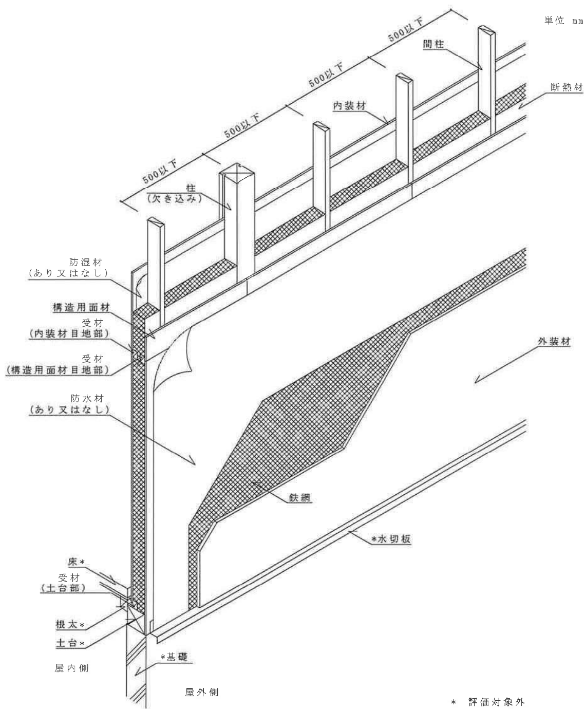
透視図
