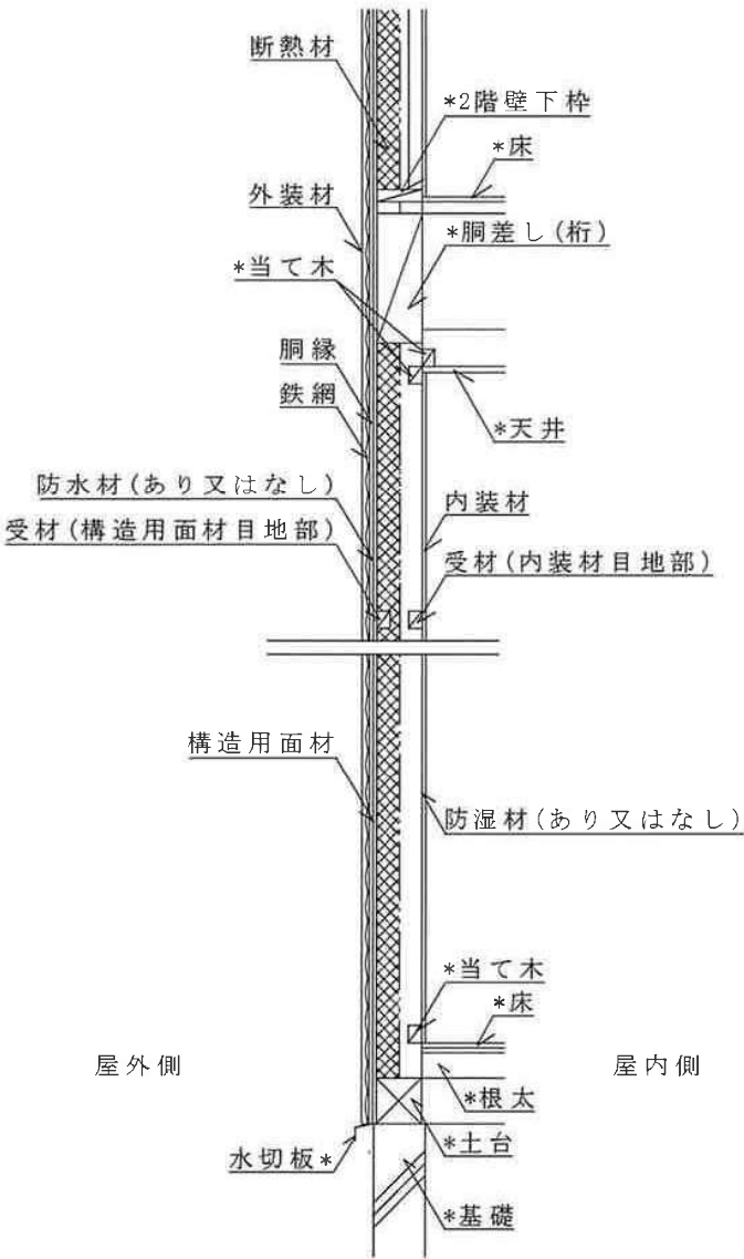
鉛直断面図
