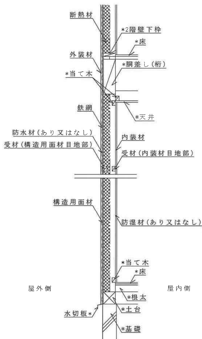
鉛直断面図
