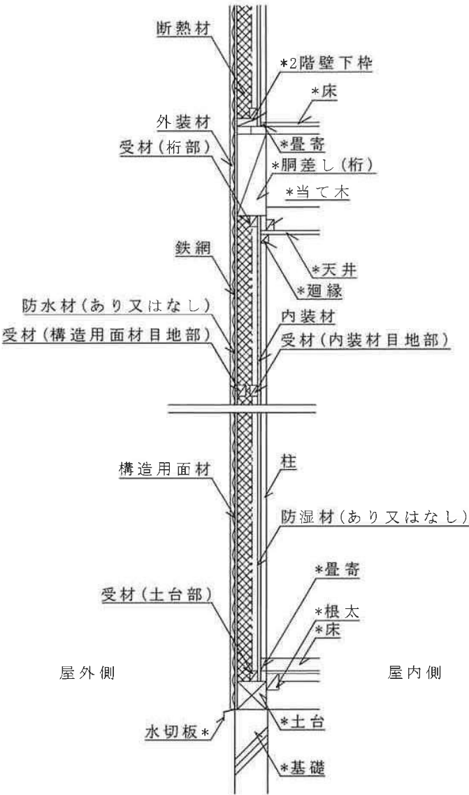
鉛直断面図
