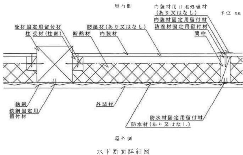
水平断面詳細図
