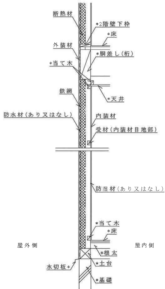
鉛直断面図
