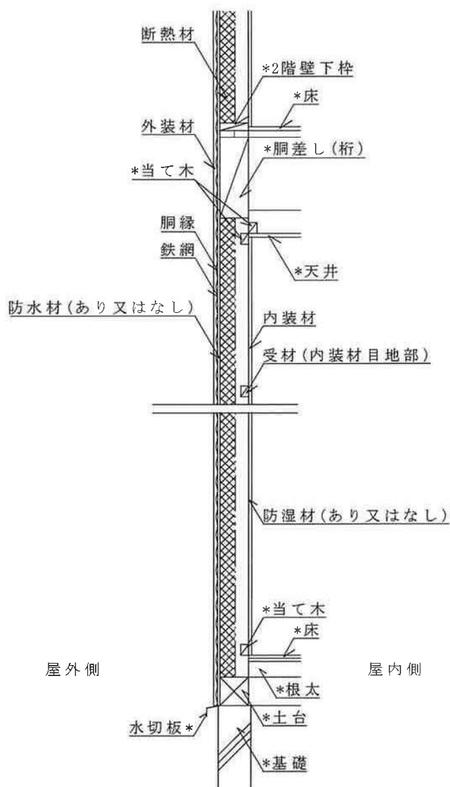
鉛直断面図
