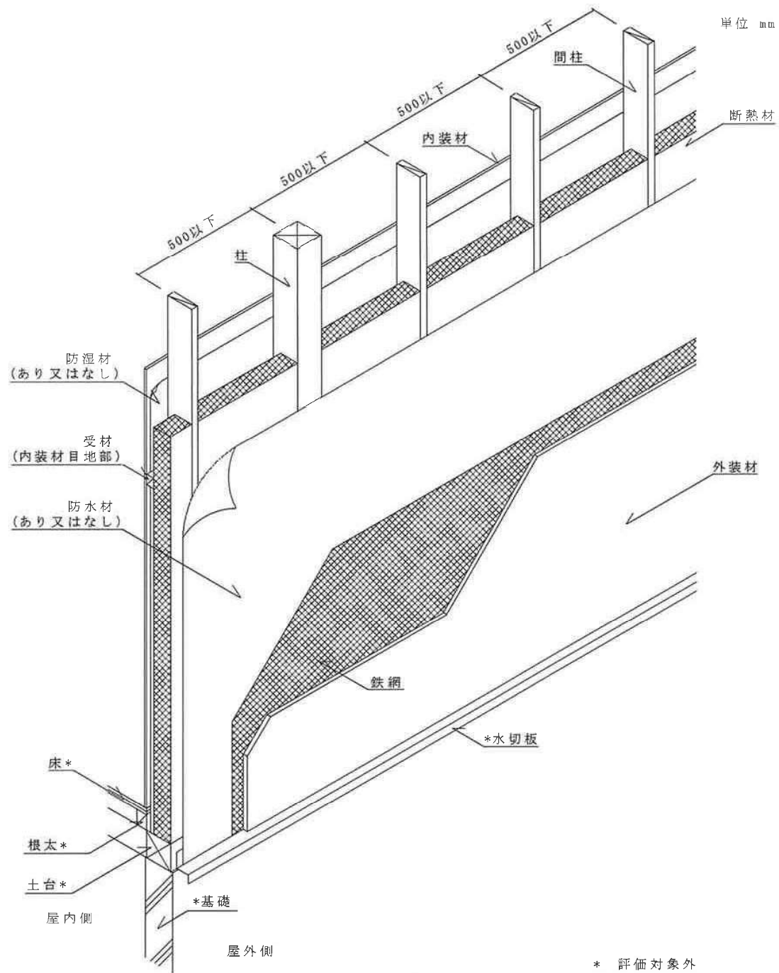
透視図
