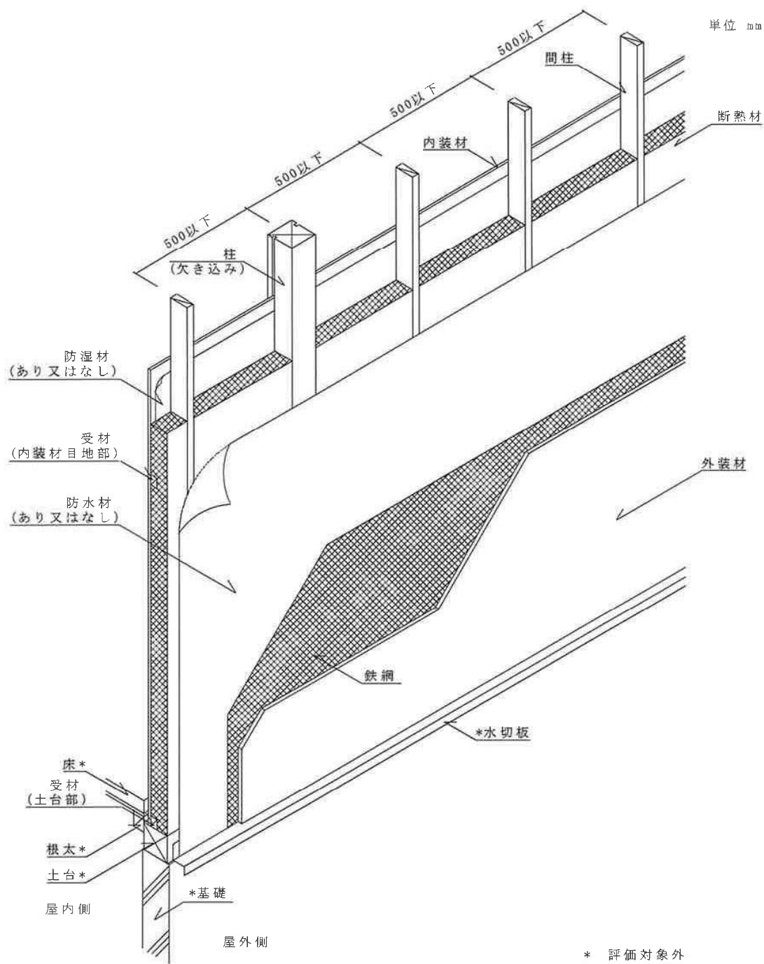
透視図
