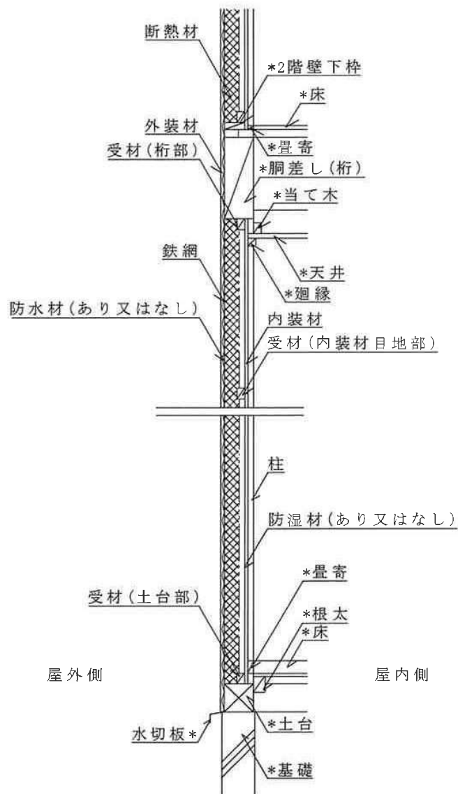
鉛直断面図
