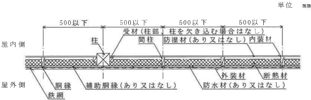
水平断面図
