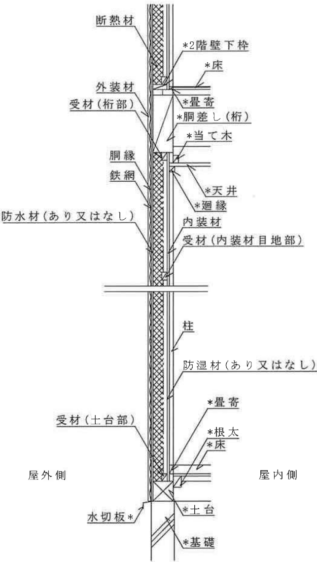
鉛直断面図
