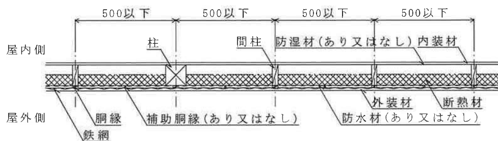
水平断面図
