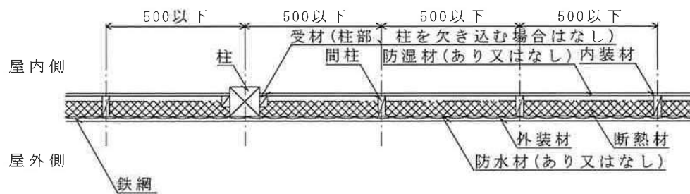
水平断面図
