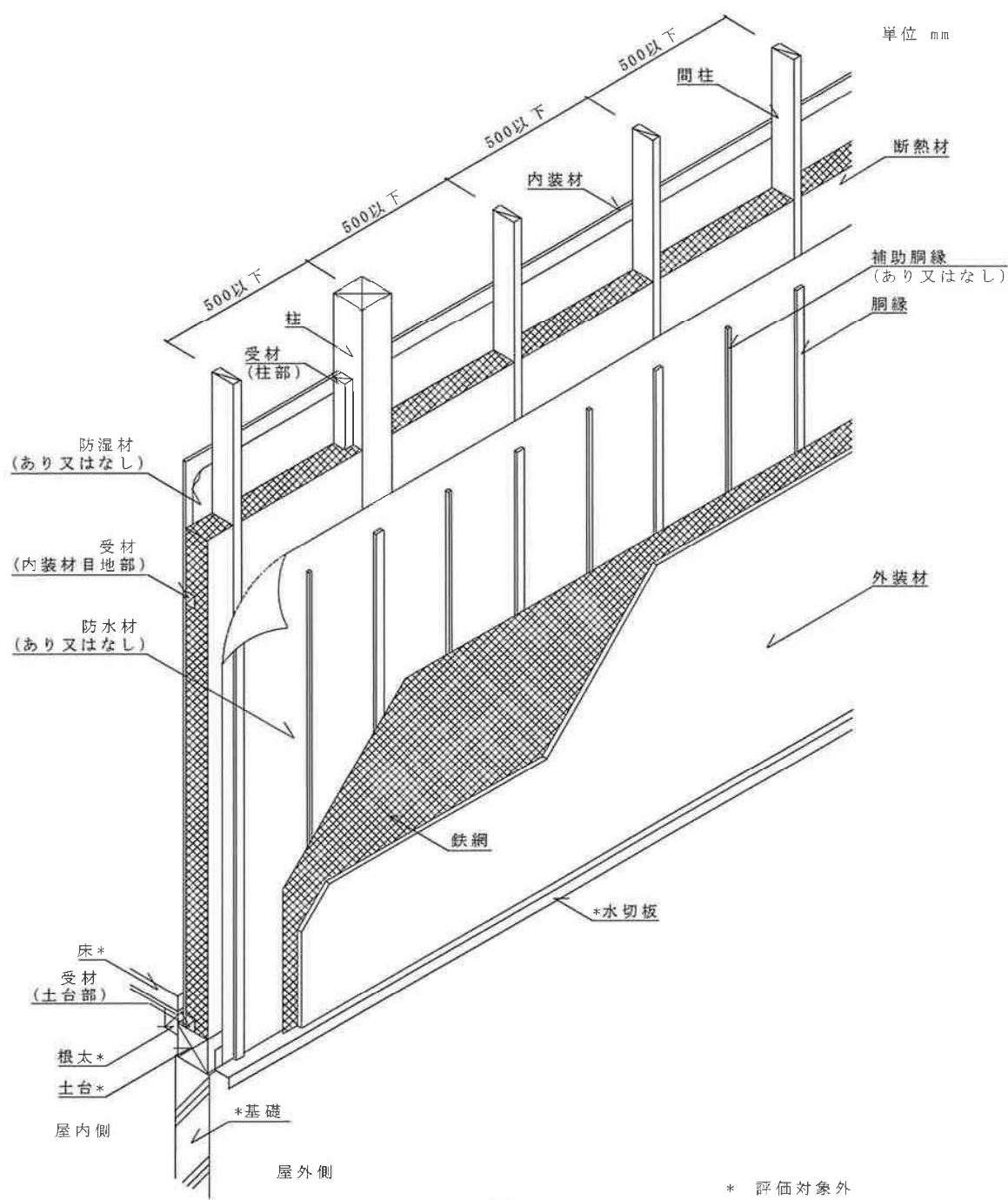
透視図
