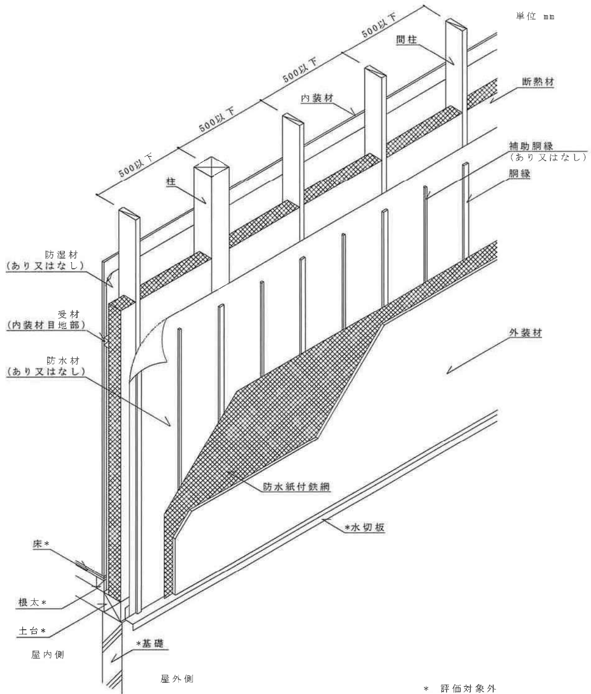
透視図
