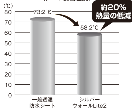
透湿防水シート遮熱性能試験 (シート裏面温度)
